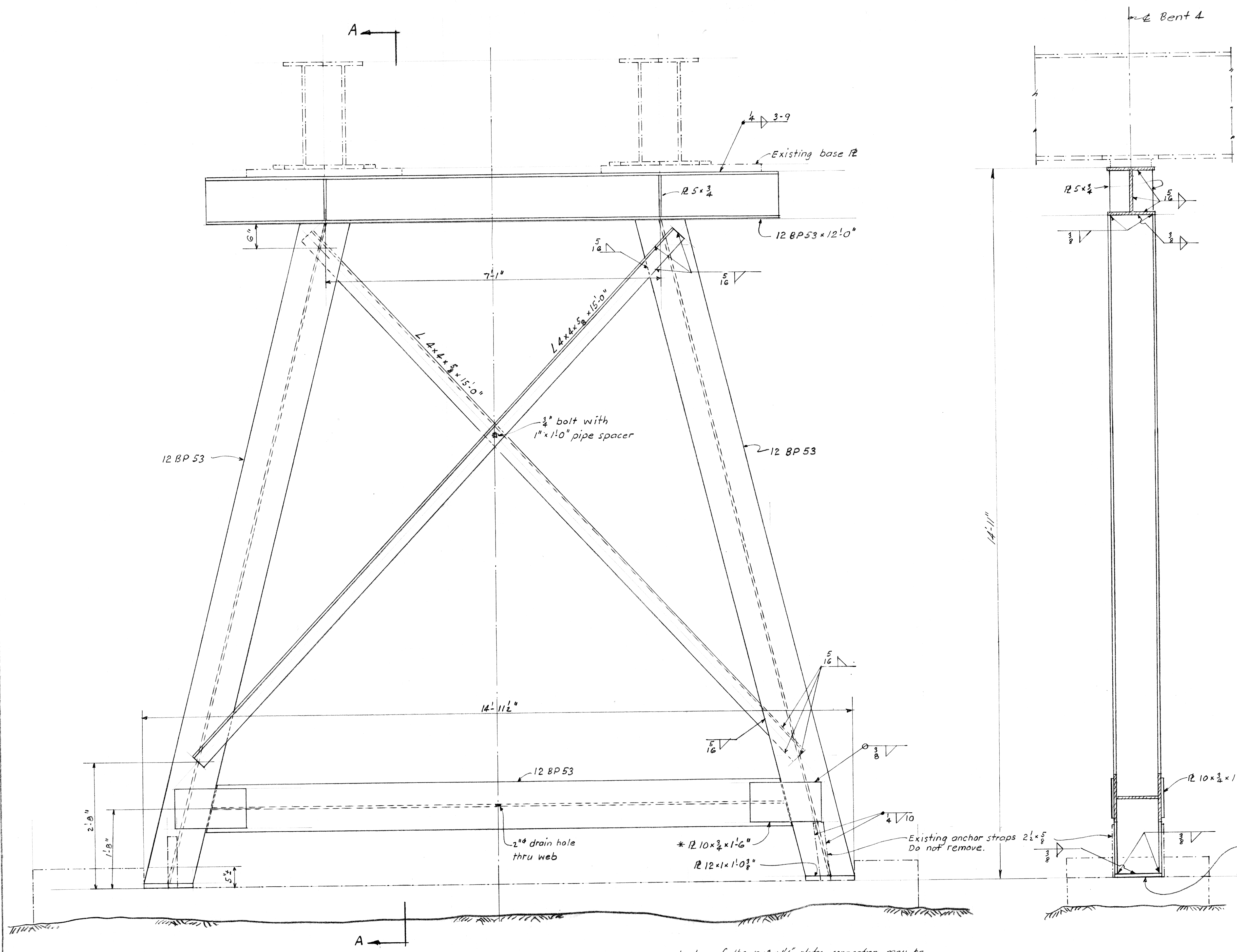
SECTION A-A
